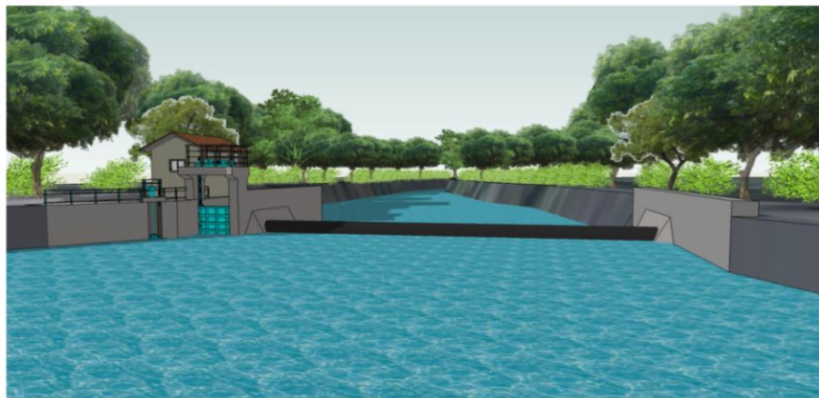
橡皮壩3D圖
